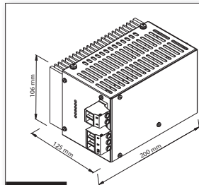
Optional DIN rail mount approx. 2.05 kg
